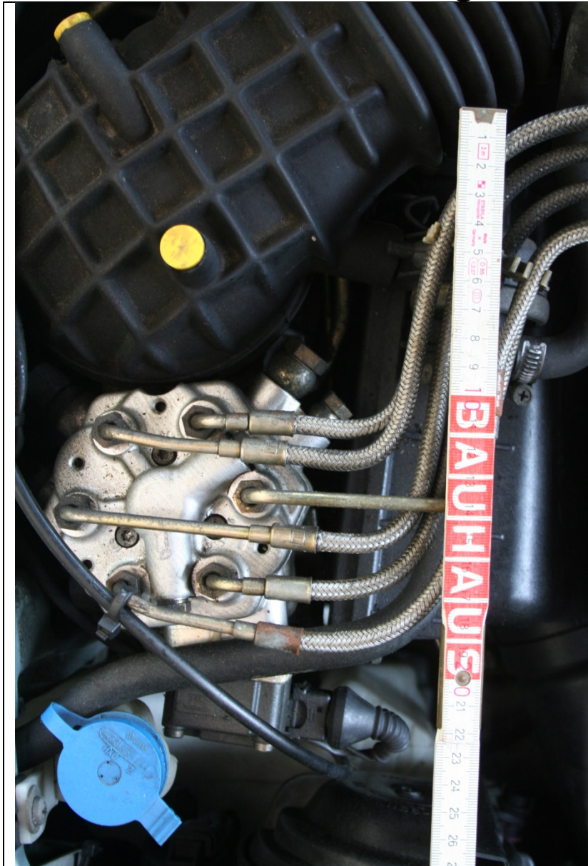
Abstand der Leitungen am mengenteiler
